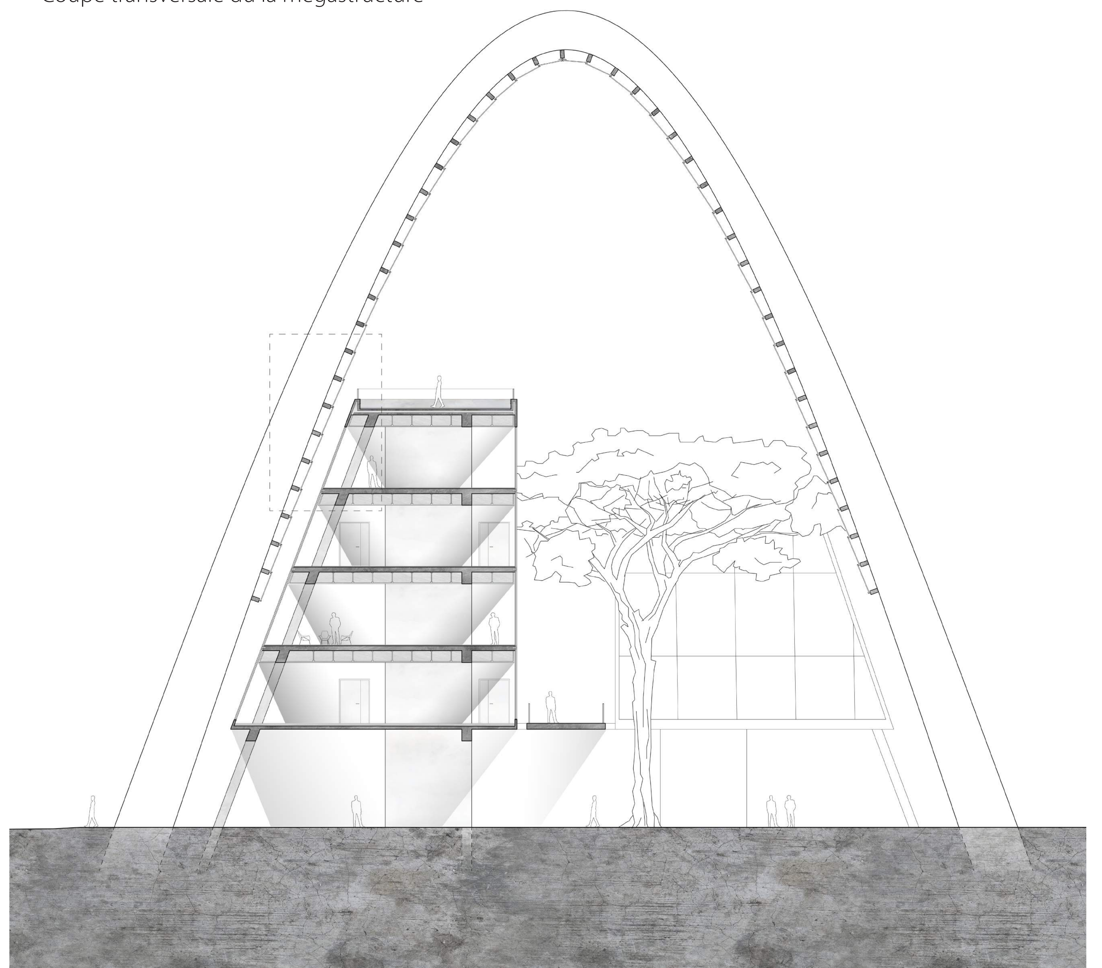
Coupe transversale de la mégastructure
