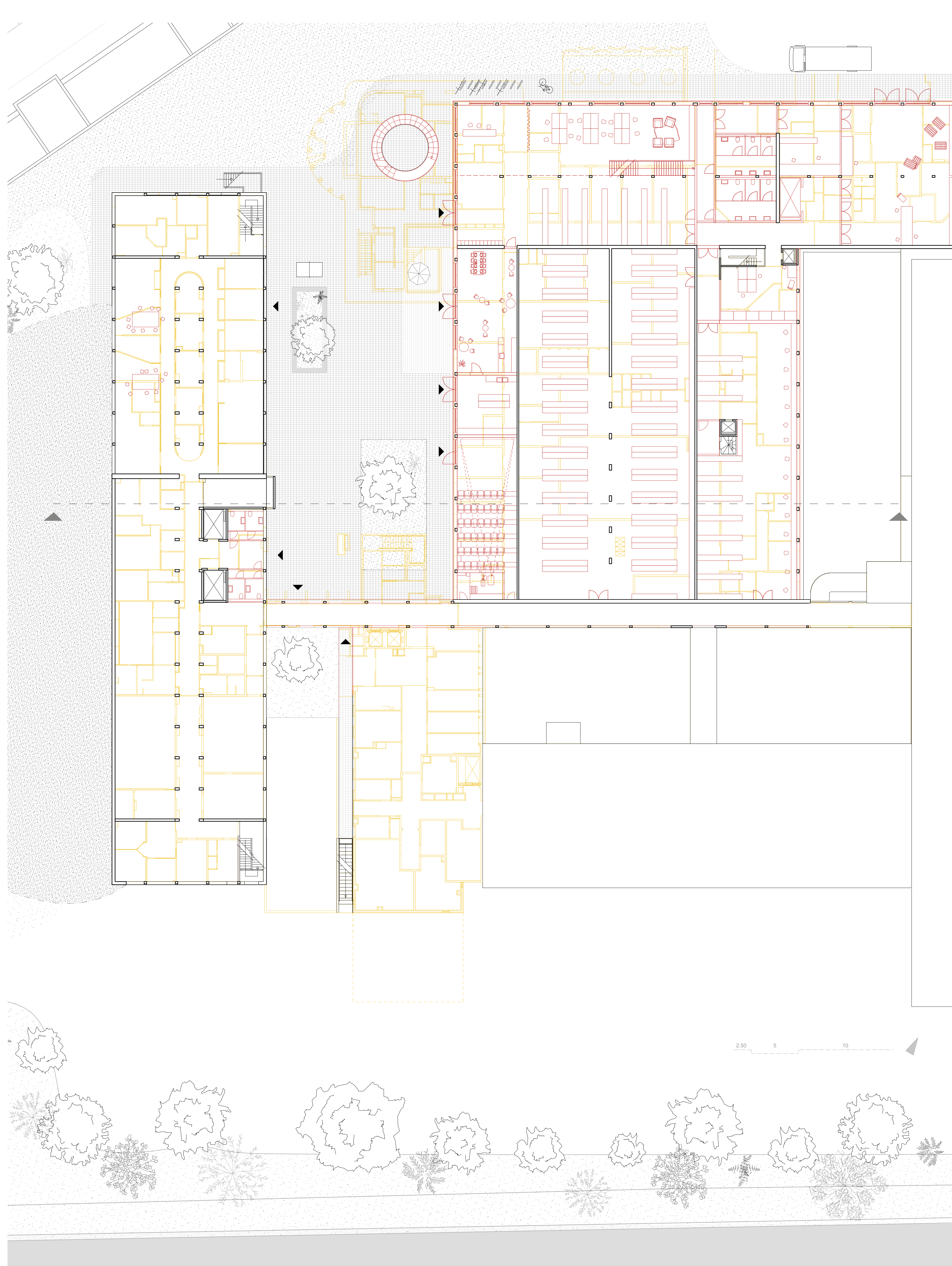
Plan du rez-de-chaussée bas et coupe 1 : 200
