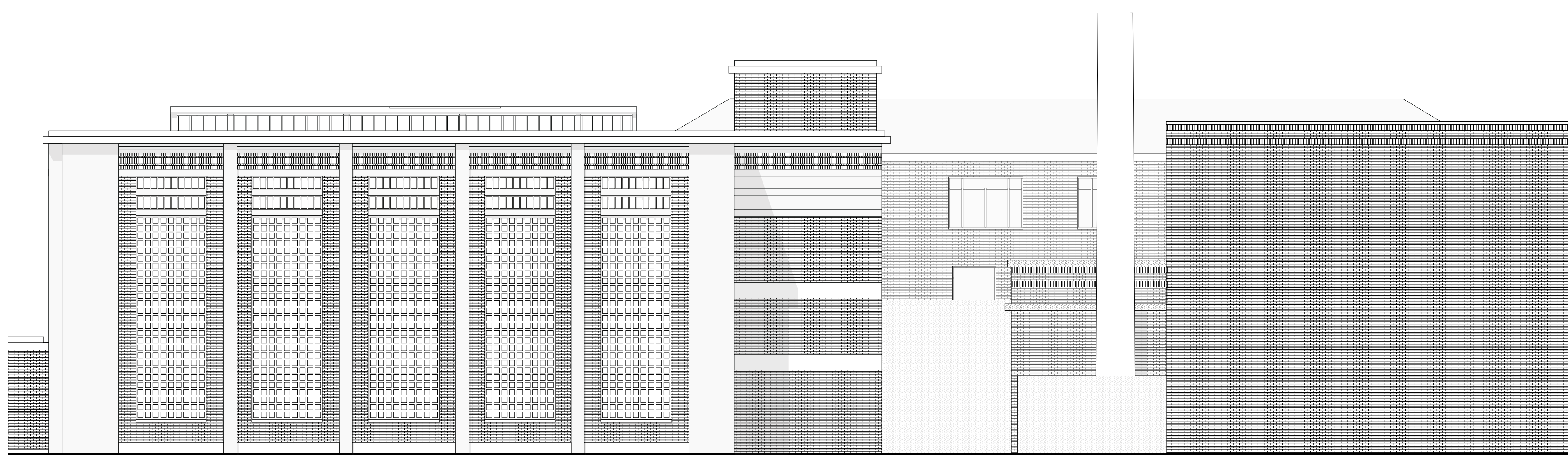
façade OUEST ancienne chaufferie, existant — 1/100
