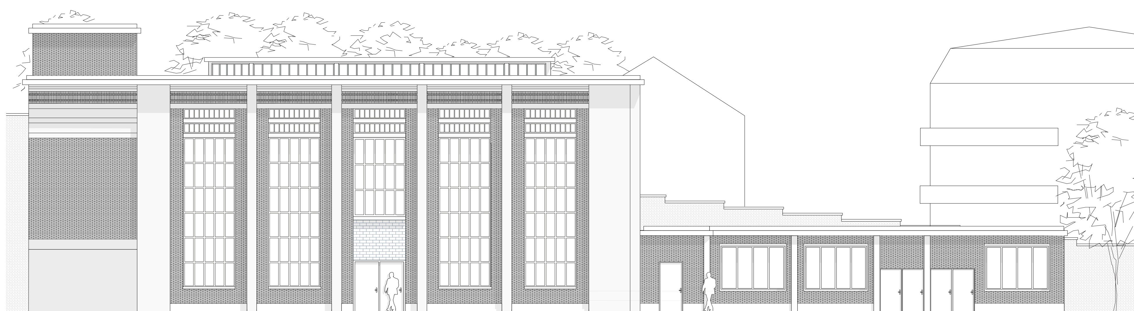
façade OUEST ancienne chaufferie, existant — 1/100
